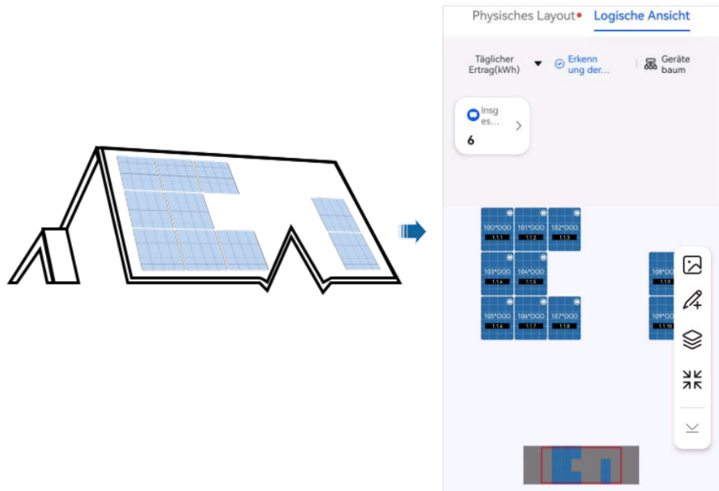
Abbildung 7-4 Anzeigen eines physikalischen Layouts in der FusionSolar-App
