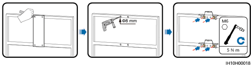
Abbildung 4-11 Anbringen der Montagehalterung
