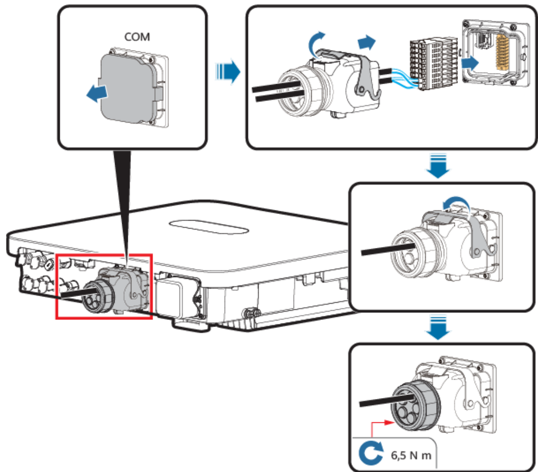
Abbildung 5-40 Sichern des Signalkabelsteckverbinders
