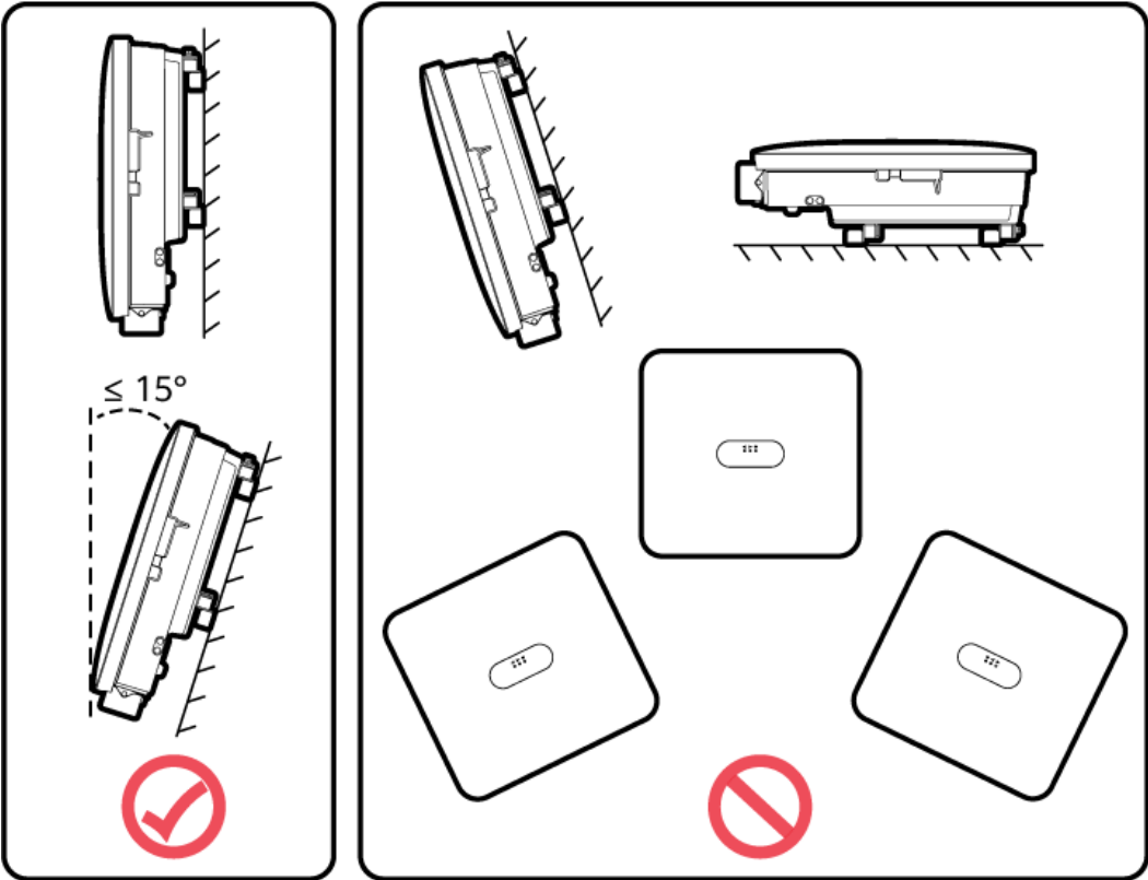
Abbildung 4-5 Installationswinkel
