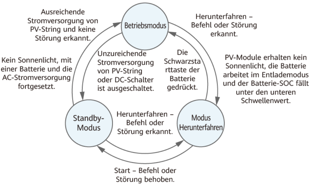
Abbildung 2-9 Arbeitsmodi
