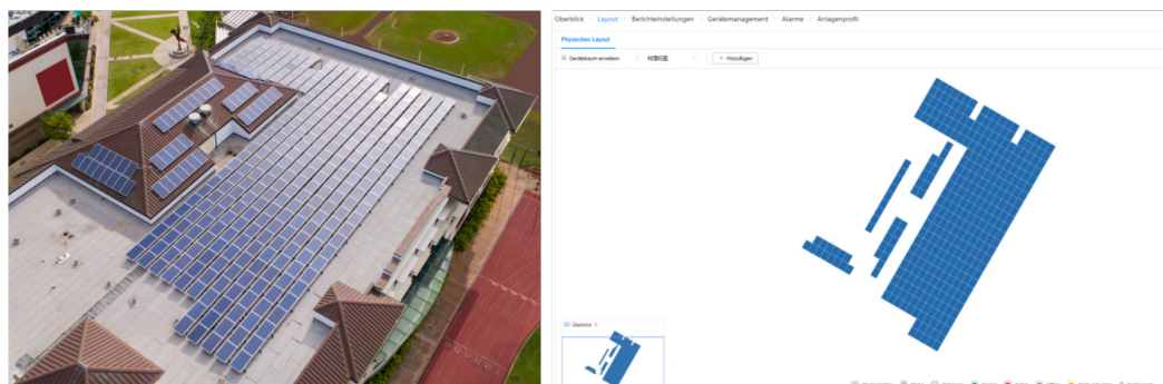
Abbildung 7-5 Anzeigen eines physikalischen Layouts im FusionSolar SmartPVMS
