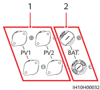
Abbildung 5-7 Klemmen
