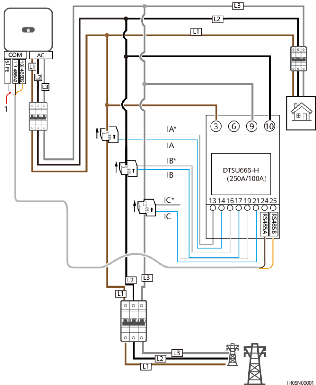
Abbildung 5-21 DTSU666-H (250 A/100 A) dreiphasige dreidrigige Kabelverbindung (Smart Dongle-Vernetzung)
